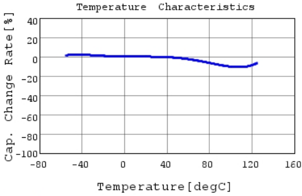
GA342DR7GF102KW02 C-Temp. capchange, DCOV, 1
