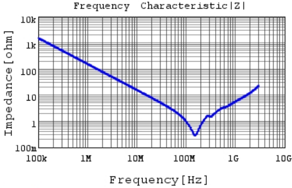
GA342DR7GF102KW02 |Z| DCOV, 25degC
