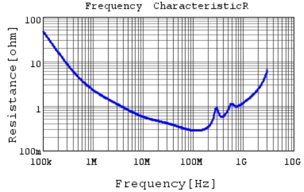
GA342DR7GF102KW02 R DCOV, 25degC
