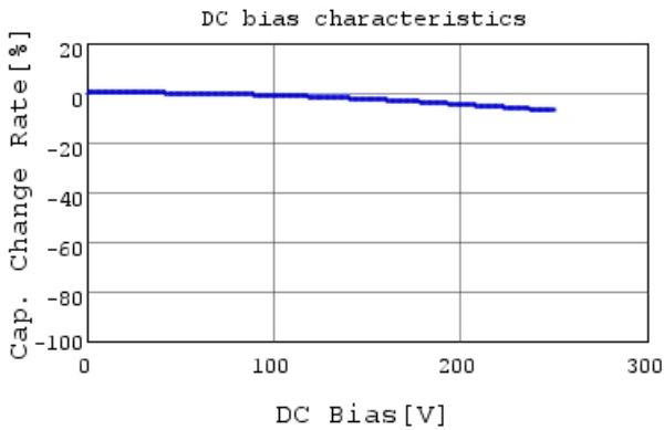
GA342DR7GF102KW02 C-DC bias capchange, 25.0c
