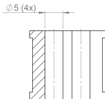
SCHNITT A-A
